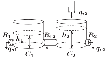
図 2: 2 タンクシステム
