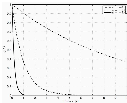
図 1: 1 次遅れ系の応答
